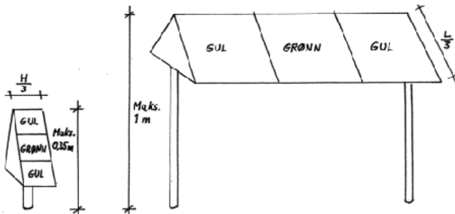
Fig. 4 Merking av lufttaksbane
