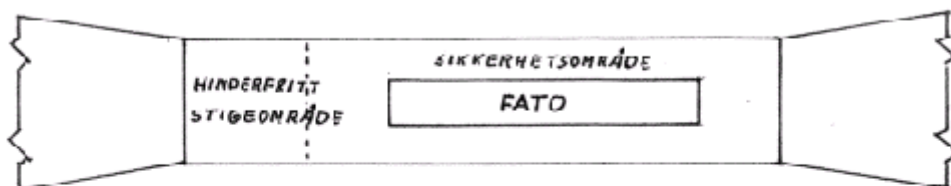
Fig 1 Sikkerhetsområde og hinderfritt stigeområde - IFR-forhold
