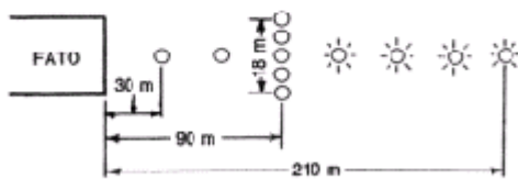
Fig. 6 INNFLYGINGSLYSANLEGG
