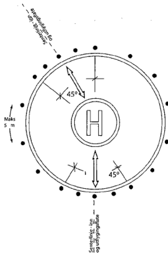
Fig. 3 Plassering av kantlys
