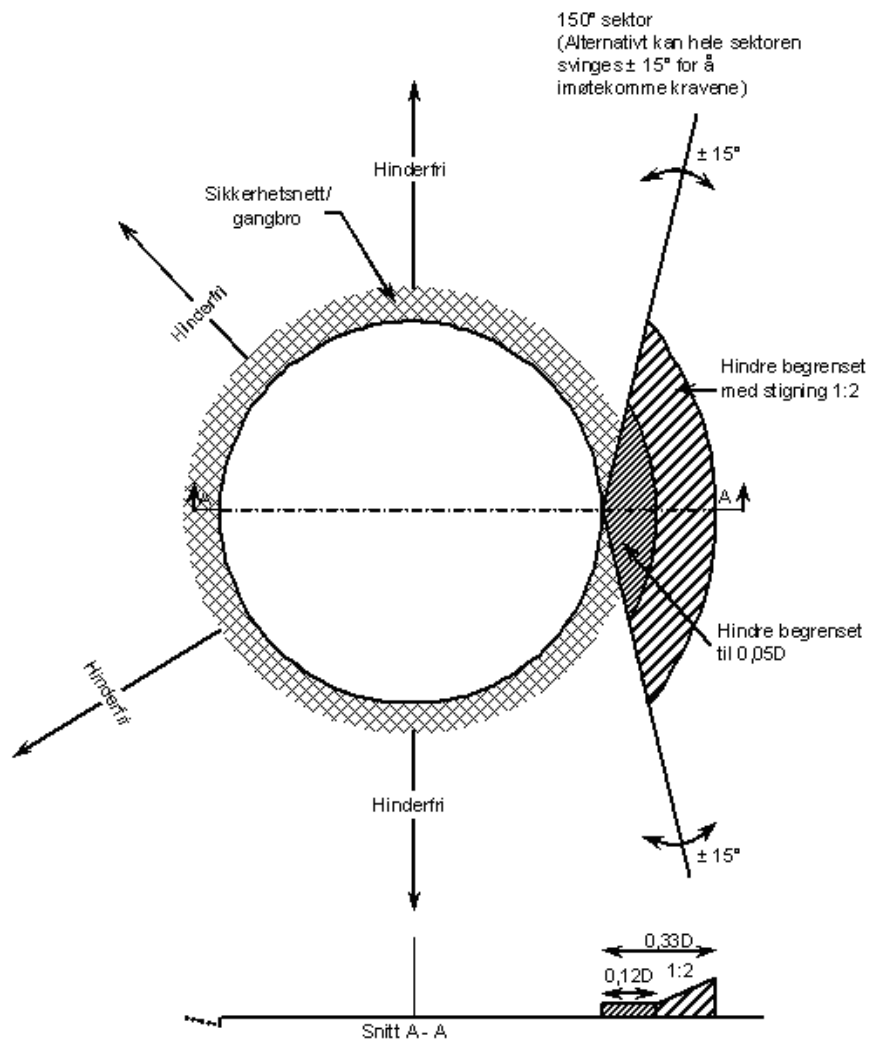
Figur 3. Hinderbegrensninger
