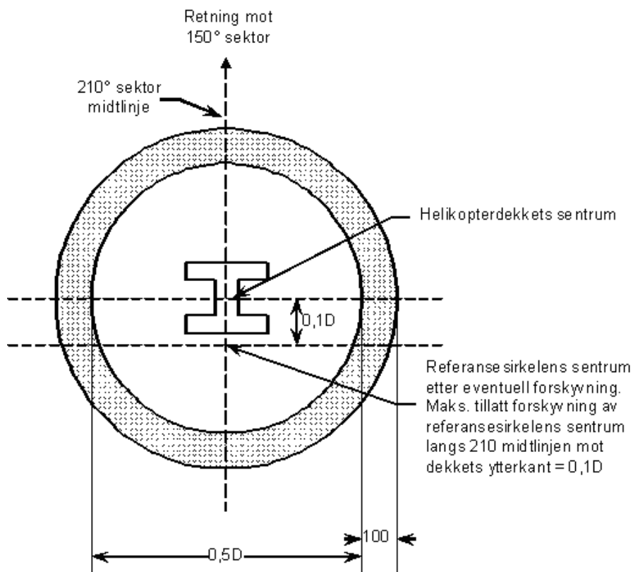
Figur 6. Referansesirkel (mål i cm)
