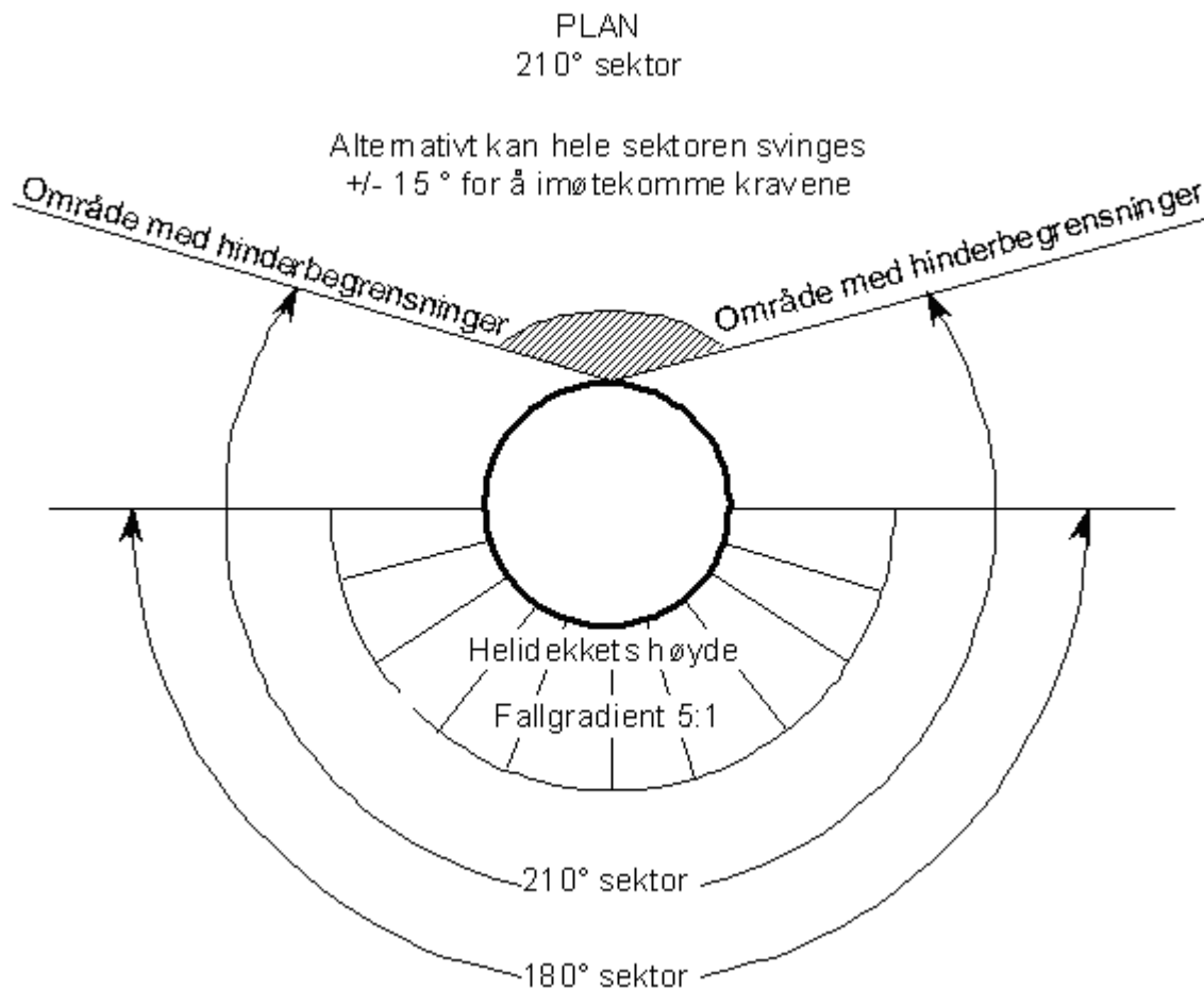
Figur 1. Hinderfri inn- og utflygingssektor, plan
