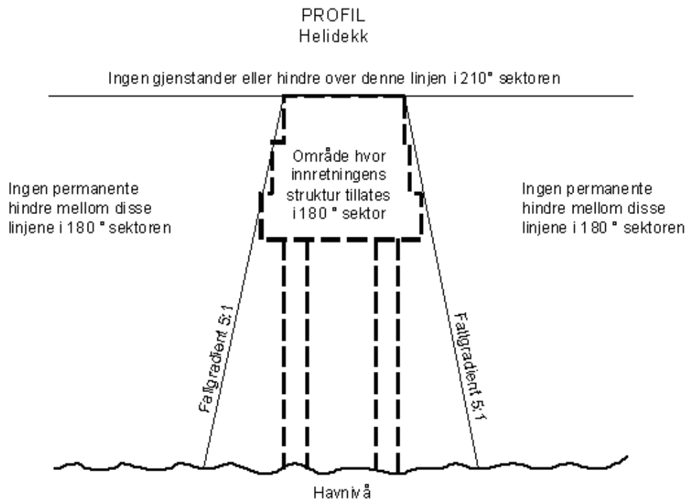
Figur 2. Hinderfri inn- og utflygingssektor, profil
