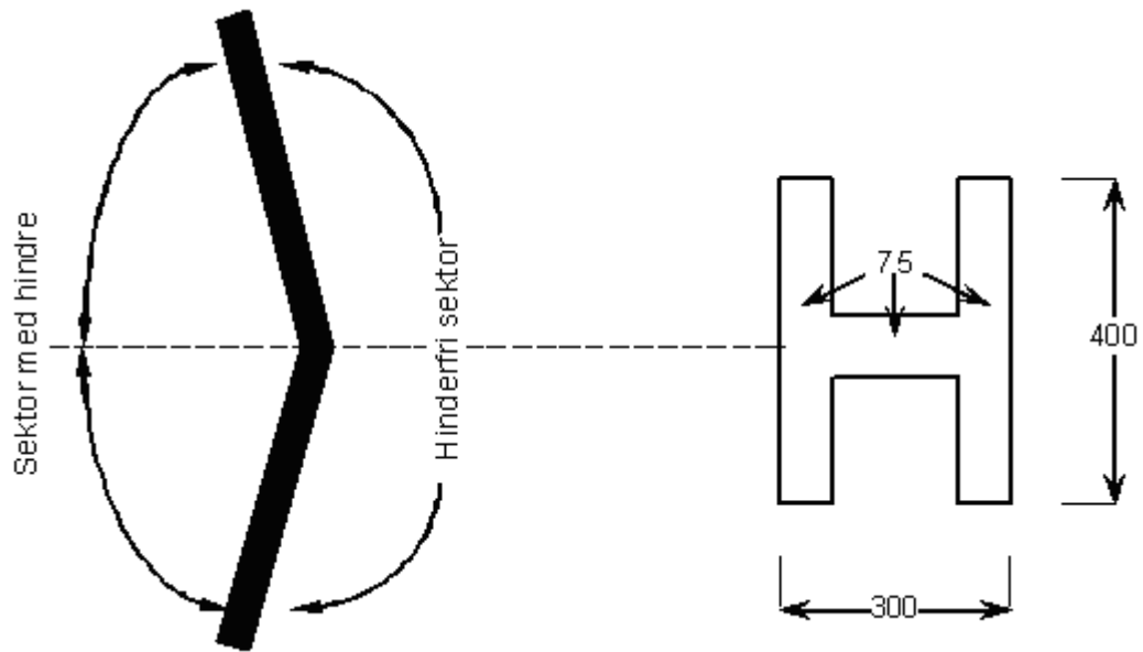
Figur 4. Identifikasjonsmerking (mål i cm)
