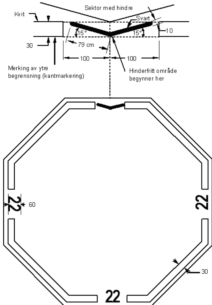
Figur 7. Merking av hinderfri sektor og D-verdi (mål i cm)
