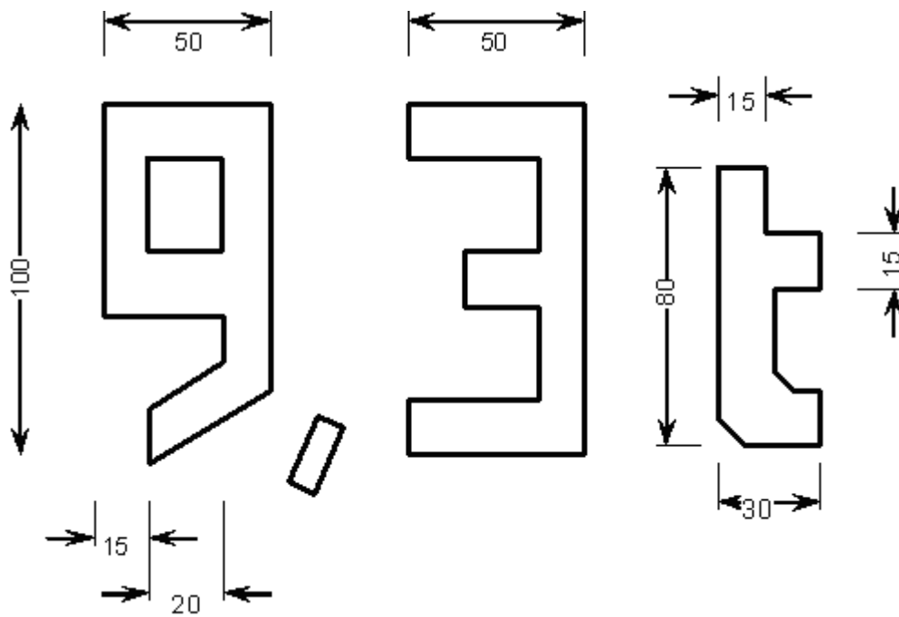
Figur 5. Merking av største tillatte masse (mål i cm)
