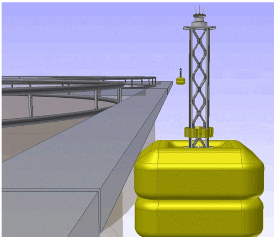
Fig. 2. Prinsippkisse av akvakulturanlegg for fisk (2).
