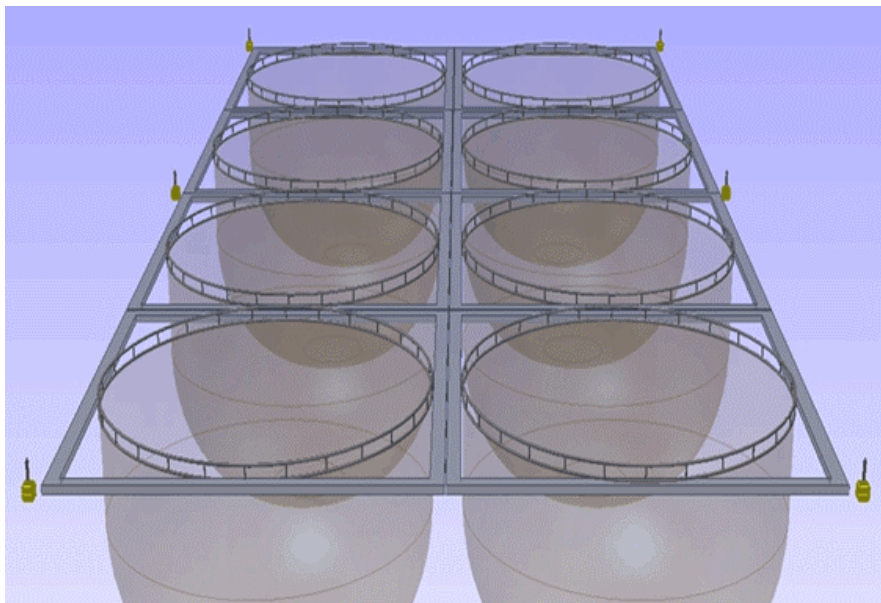
Fig. 1. Prinsippkisse av akvakulturanlegg for fisk (1).
